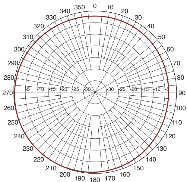
5400MHz - AZ
