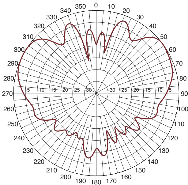
2450MHz - EL PHI90
