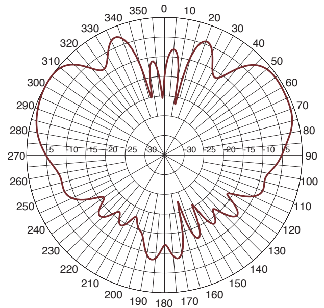
2450MHz - EL PHI0
