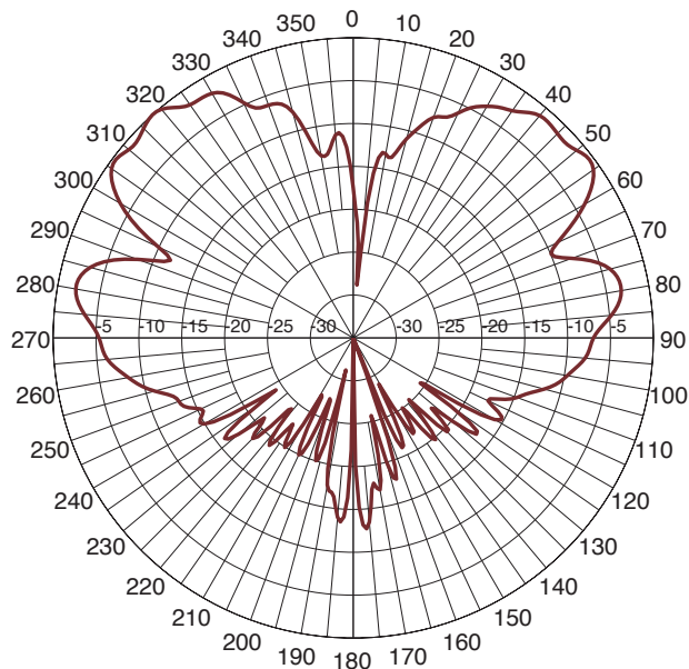
5400MHz - EL PHI0
